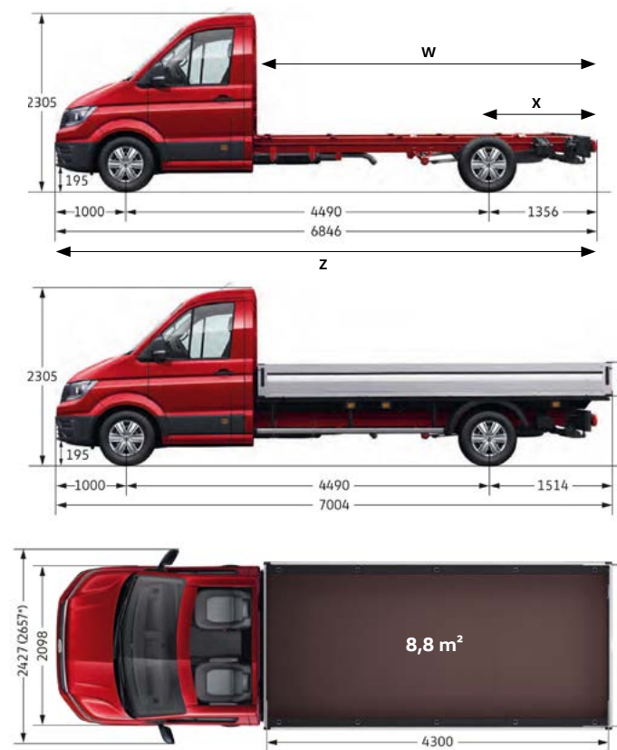
L4SC (Châssis nu + plateau)
